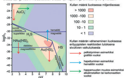
Kuva 3. Kullan liukoisuus erilaisina kompleksioneina fluidiin sen happamuuden (pH) ja hapetus-tilan ( \log fO_2 ) mukaan. Nuolet osoittavat, kuinka kulan liukoisuus laskee nopeasti miljoonasosasta miljardiosaan fluidin koostumuksen muuttuessa erilaisten ulkoisten tekijöiden vaikutuksesta. Mukailtu Hayashilta ja Ohmotolta (1991).
